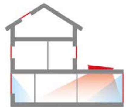
Uitbouw met lichtstraat. Comfortabele ruimte, ideaal daglicht
