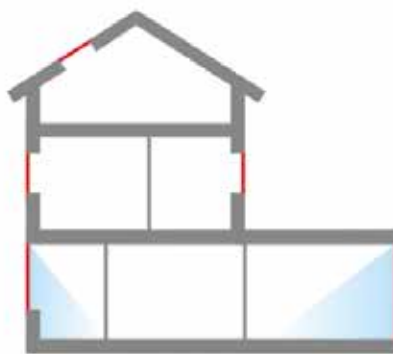
Standaard uitbouw. Meer ruimte, minder daglicht
